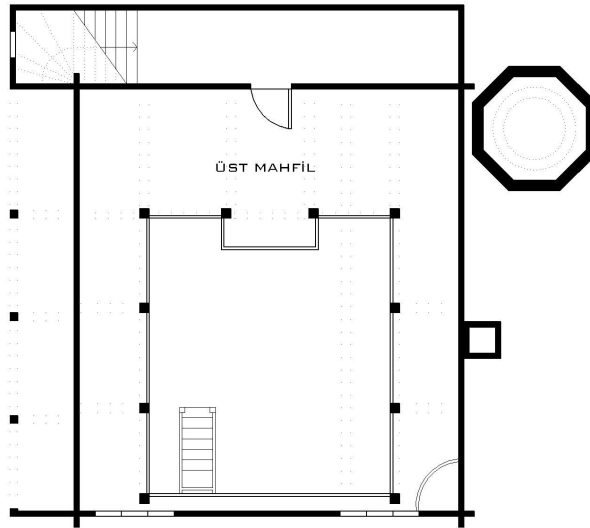
Şekil 3. Filak Mahallesi Ahşap Cami Üst Kat Plan Şeması
