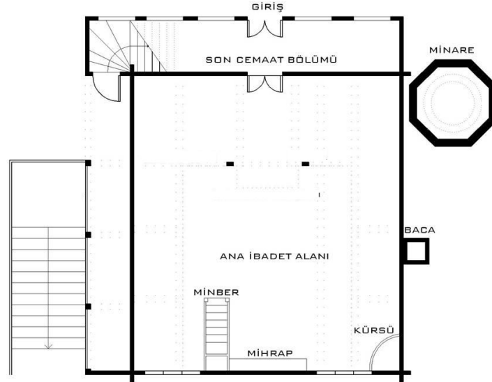
Şekil 2. Filak Mahallesi Ahşap Cami Zemin Kat Plan Şeması
