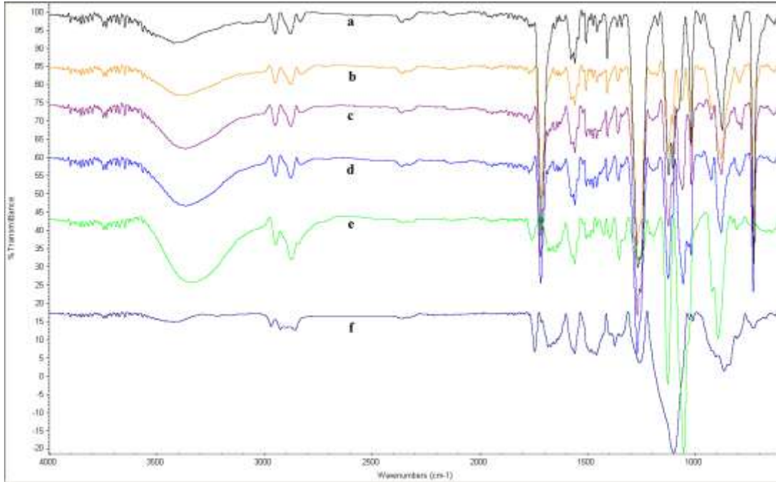
Şekil 4. FTIR sonuçları a: DEG10, b: DEG20, c: DEG25, d: DEG 30 e: Dietilen Glikol, f: ticari poliöl
