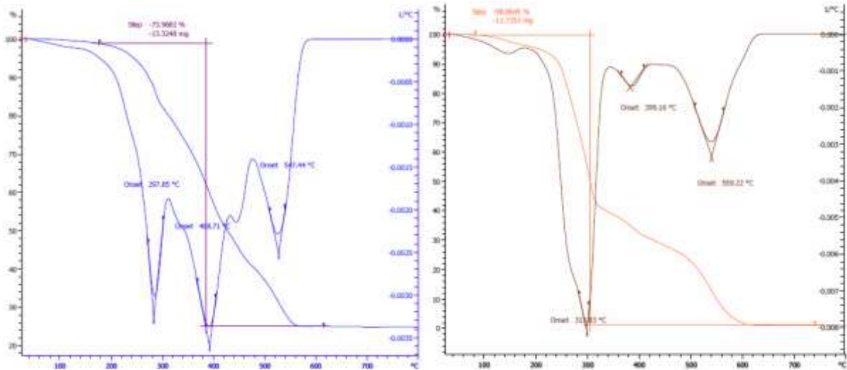
Şekil 6. Ticari poliüretan ve balyalama iplerinden elde edilen ürün ile üretilen poliüretanın TGA analizi.
